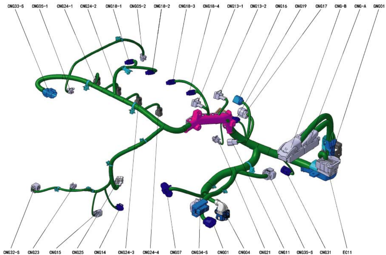
控制线束(1)
